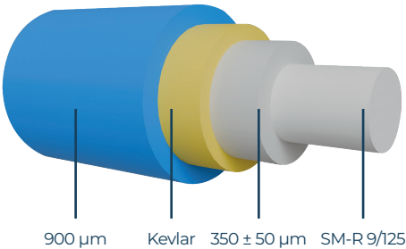
DETTAGLIO CAVO PICOBREAKOUT (altre colorazioni secondo tabella)
