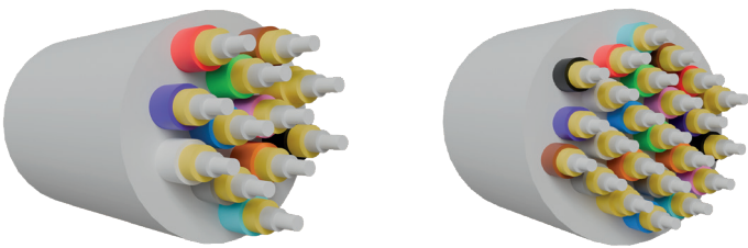
DETTAGLIO CAVO PICOBREAKOUT (altre colorazioni secondo tabella)
